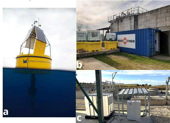
Impianti pilota per la rimozione e il monitoraggio di CoEC presso: (a) Cipro (Limassol), (b) Italia (Torino, Brandizzo) e (c) Spagna (San Esteban De Litera).
